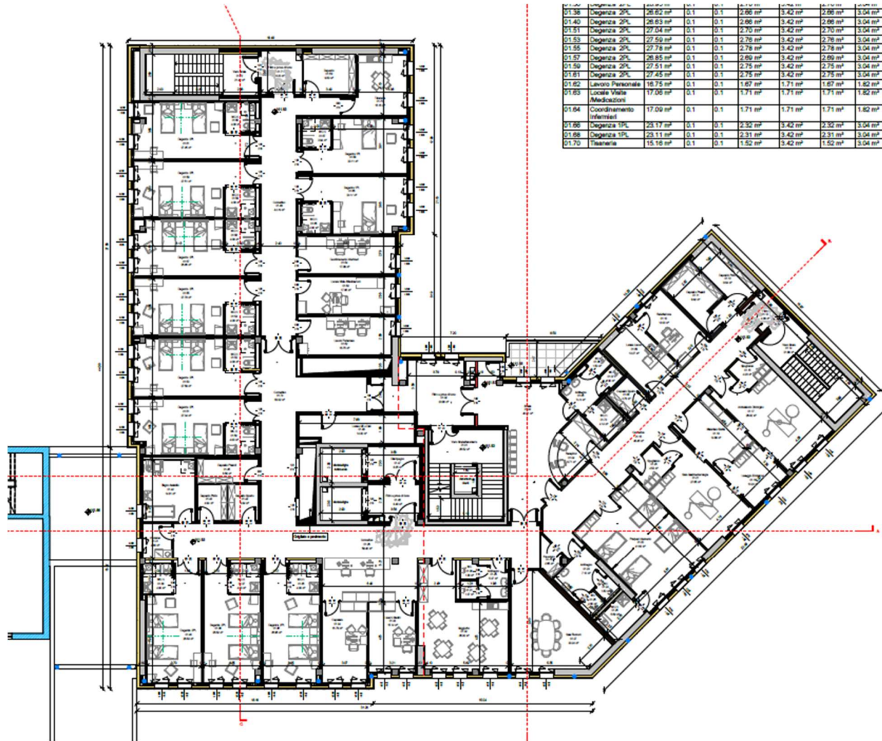
Pianta Piano primo intervento OdC
