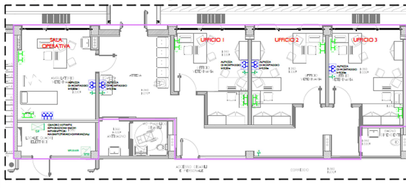
Pianta di progetto
