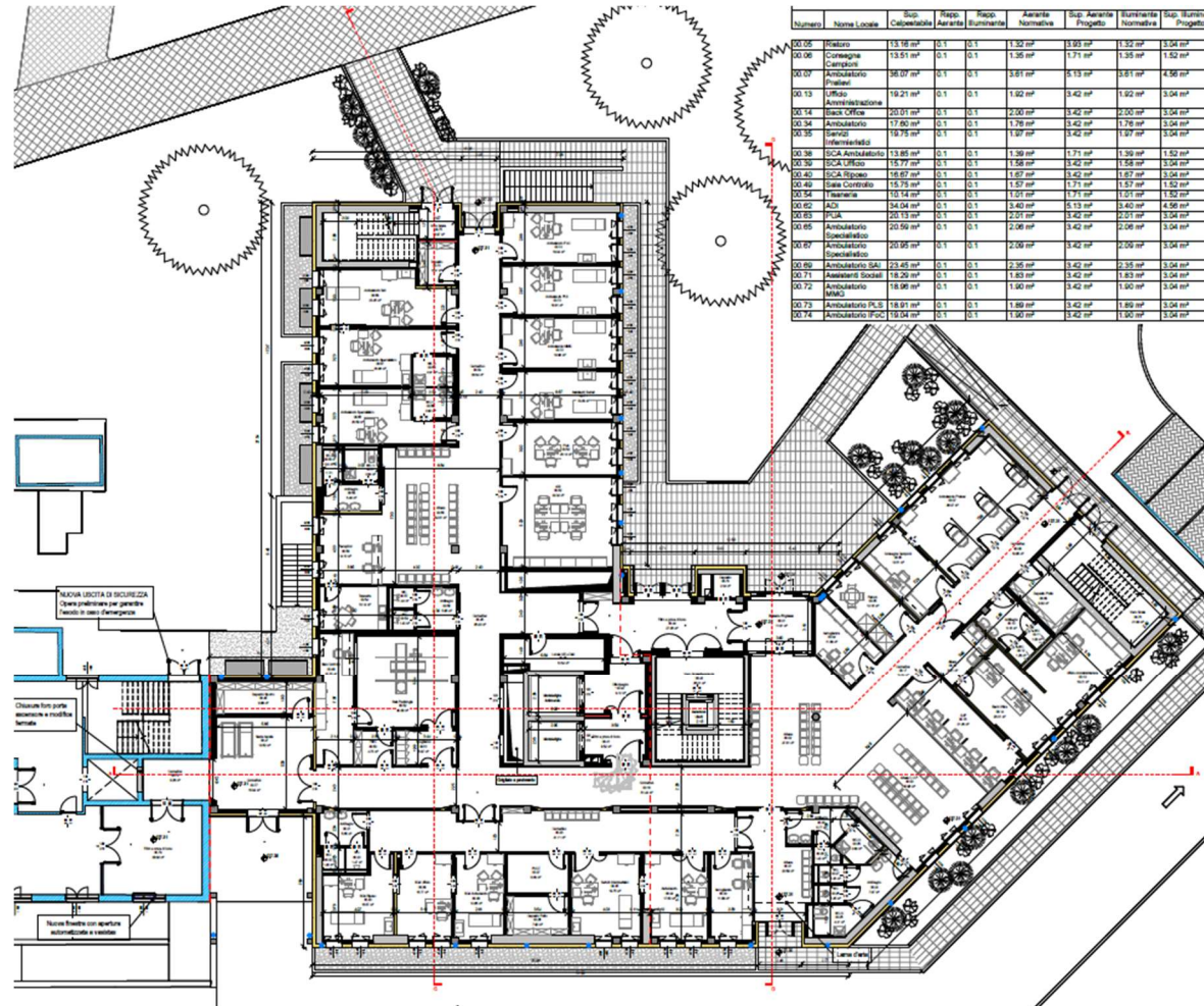
Pianta piano Terra intervento CdC
